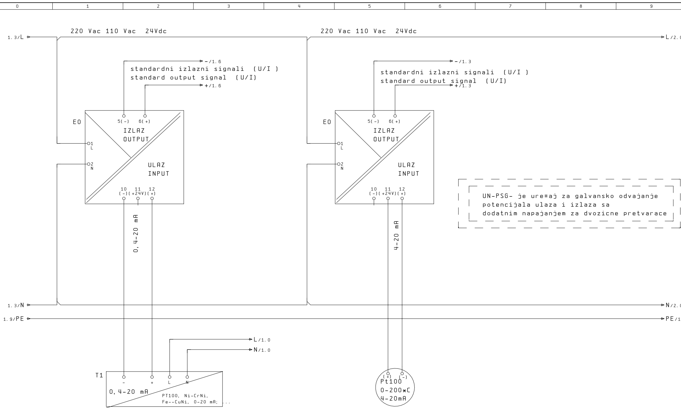
SPOJ CETVEROZICNOG PRETVARACA NA GALVANSKO ODVAJANJE POTENCIJALA SIGNALA
