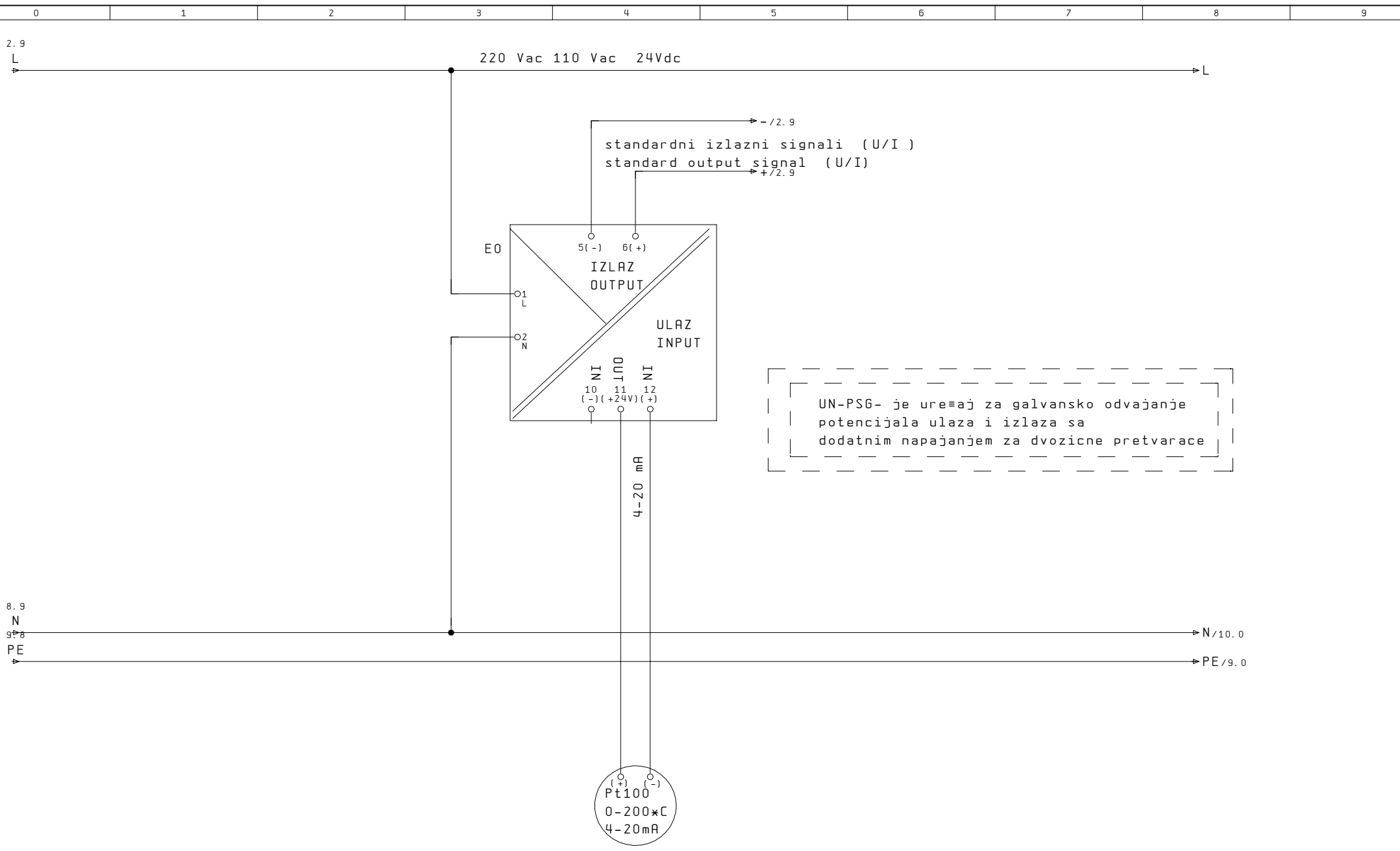
SPOJ DVOZICNOG PRETVARACA NA GALVANSKO ODVAJANJE POTENCIJALA SIGNALA
